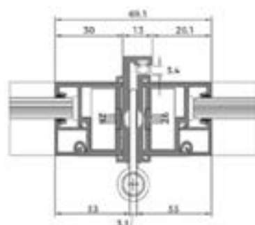
Detalle unión bisagra perfil
