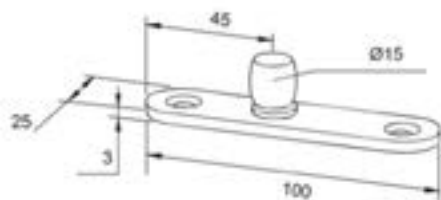
Pivote
