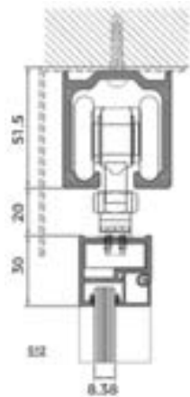
Detalle guía
