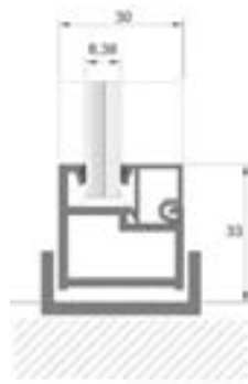
Detalle guiador suelo
