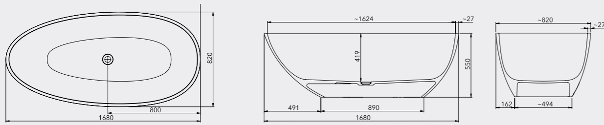
STELLA (SIFÓN SIN REBOSADERO INCLUIDO)
