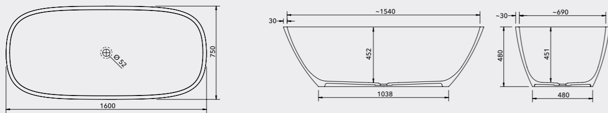
SILK (SIFÓN SIN REBOSADERO INCLUIDO)
