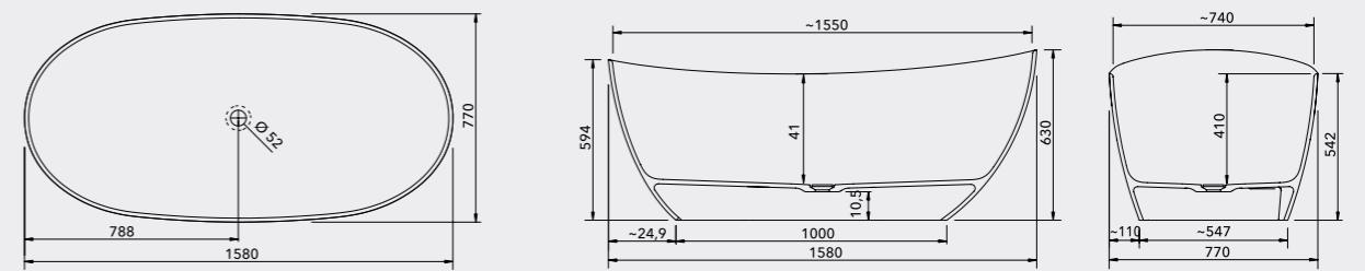
BECCA (SIFÓN SIN REBOSADERO INCLUIDO)
