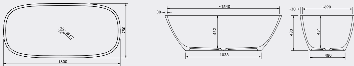
DAFNE (SIFÓN SIN REBOSADERO INCLUIDO) (TAPA DE VÁLVULA EN RESINA)
